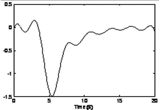
图 6 无功功率变化曲线
