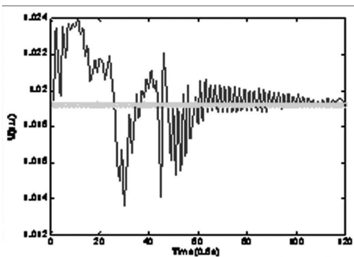
图 7 母线电压波动情况
