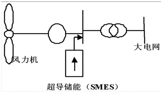
图 3 采用 SMES 的风力场系统
