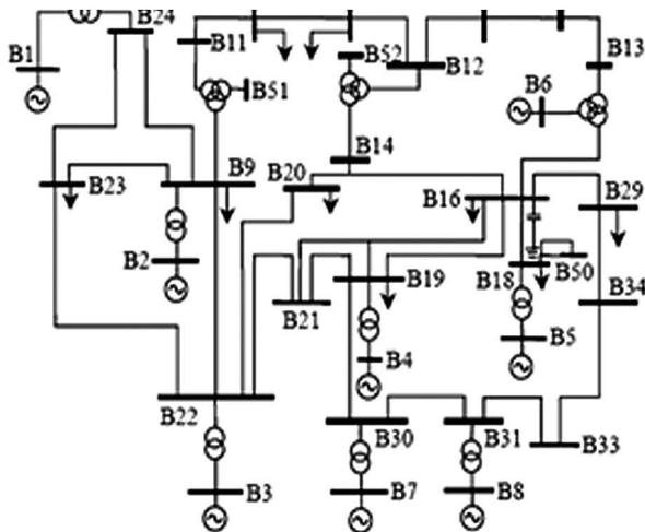
图 4 EPR1-36 节点系统
