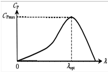
图 1 C_p 与 \lambda 的关系
