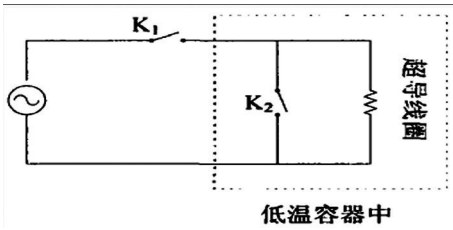
图 2 超导储能装置原理图
