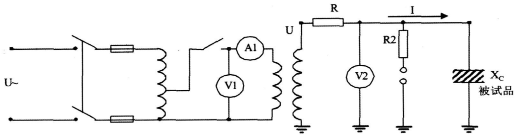
图 1 交流耐压试验接线图
