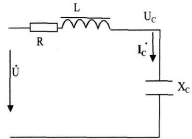
图 3 串联谐振耐压试验接线简图
